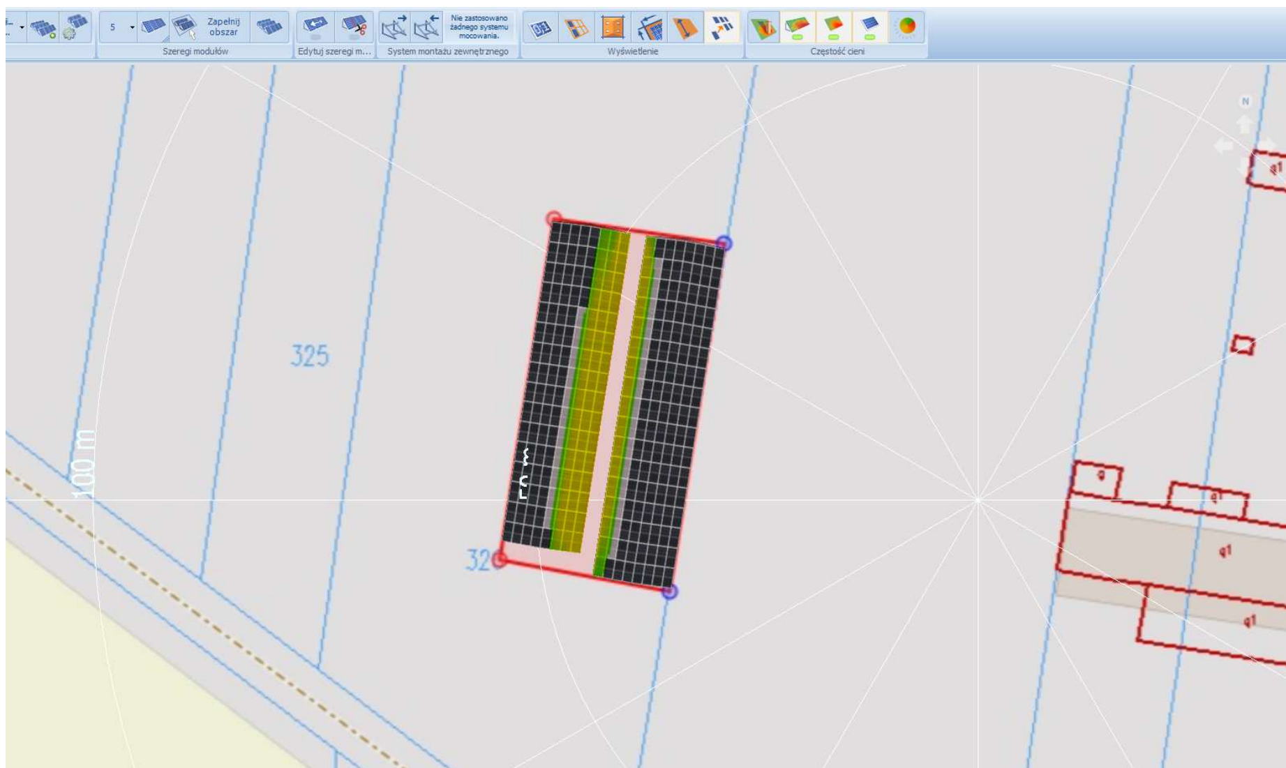
Panele Ja Solar JAM72D30 540-565/GB 264 szt. 149,16 kW działka 750 m 2
